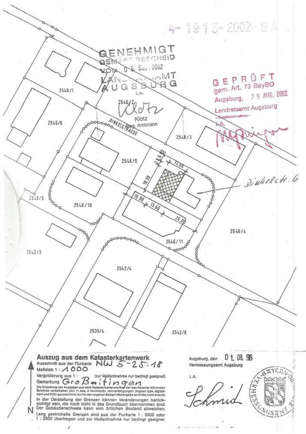
Lageplan
